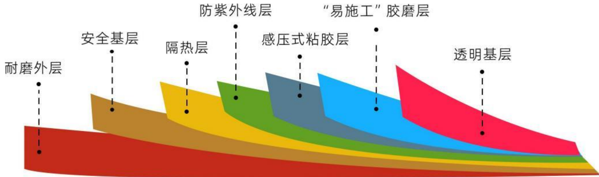
七色光®隔热膜结构图
